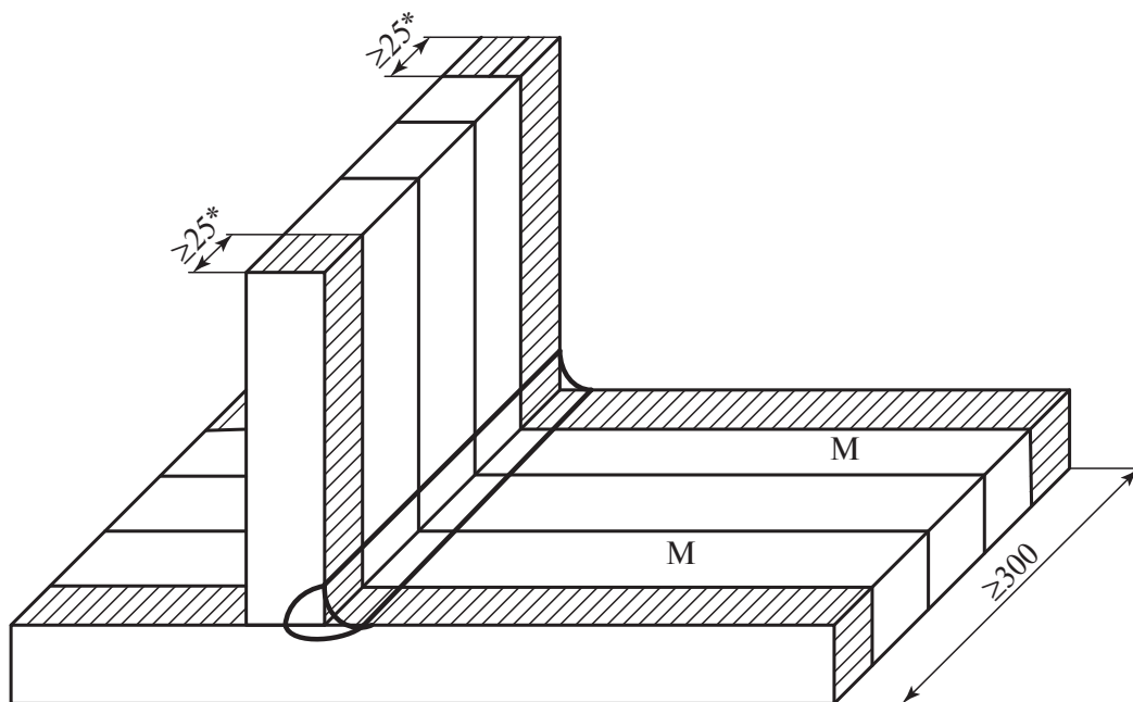
Рис. 11.15. Схема вырезки образцов из контрольных тавровых сварных соединений листов (*металл конечных участков шва, подлежащих удалению):
